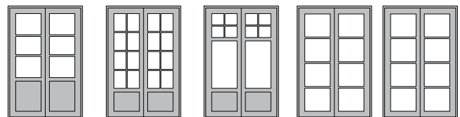
Exempel på post- och spröjsindelningar för TKDB-2 och TKDG-2.
