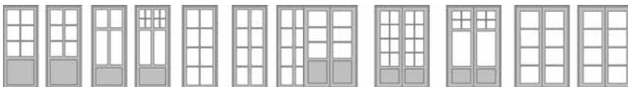
Exempel på post- och spröjsindelningar för FDBC, FDGC, FDBC-2, FDGC-2
